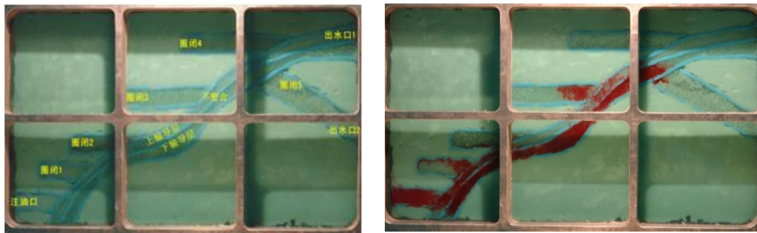
不整合纵向结构控藏机理物理模拟
