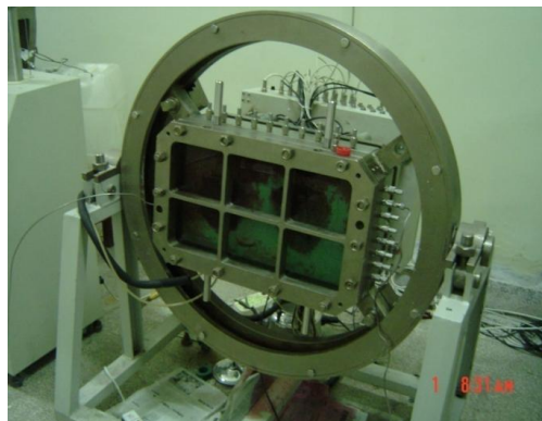
油气运聚静态模拟器
